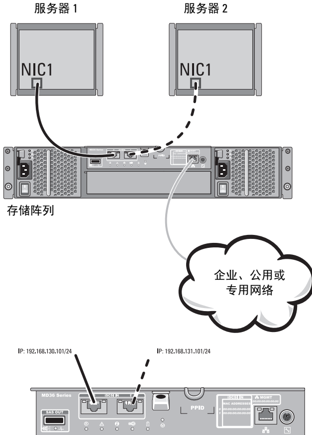
图 2-1. 两台主机连接到单个控制器
