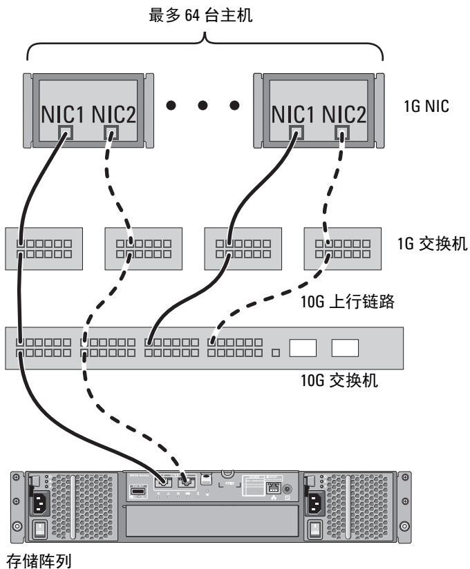
图 2-8. 64 台服务器连接到单个 RAID 控制器
