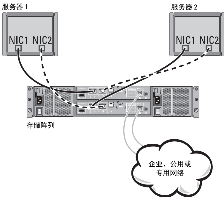
图 2-4. 两台主机连接到两个控制器
