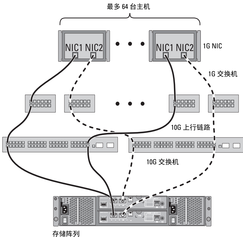
图 2-9. 64 台服务器连接到两个 RAID 控制器
