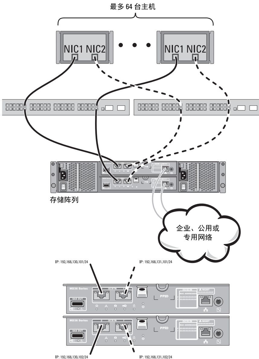
图 2-7. 64 台服务器连接到单个控制器
