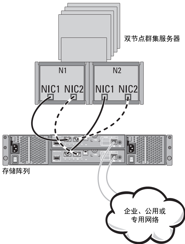
图 2-5. 双控制器配置中两台连接的主机
