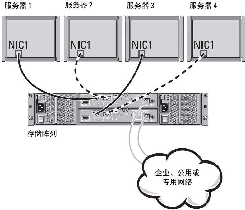
图 2-3. 双控制器配置中的四台主机
