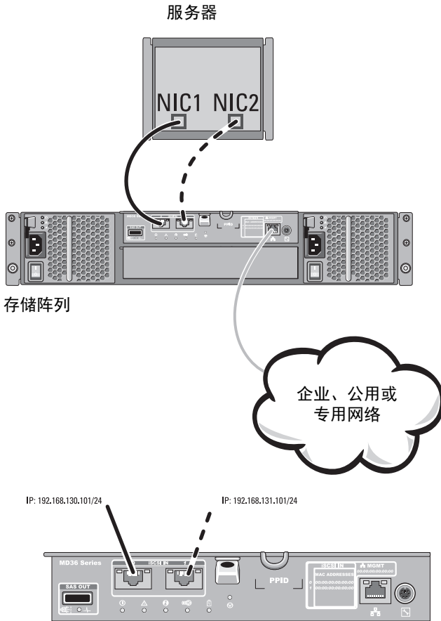
图 2-2. 连接到单个控制器的一台主机
